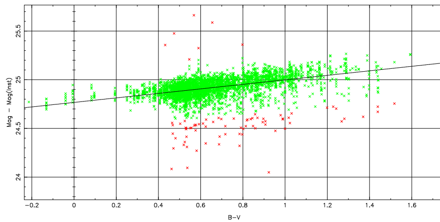
1 parameter fit: \text{Mag}-\text{Mag}(\text{Inst}) = 24.76 \pm 0.02 + (-0.22 \pm 0.00) \text{airmass} + (0.25 \pm 0.00) \text{color}
