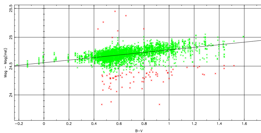
2 parameter fit: \text{Mag}-\text{Mag}(\text{Inst}) = 24.77 \pm 0.05 + (-0.22 \pm 0.00) \text{airmass} + (0.23 \pm 0.00) \text{color}
