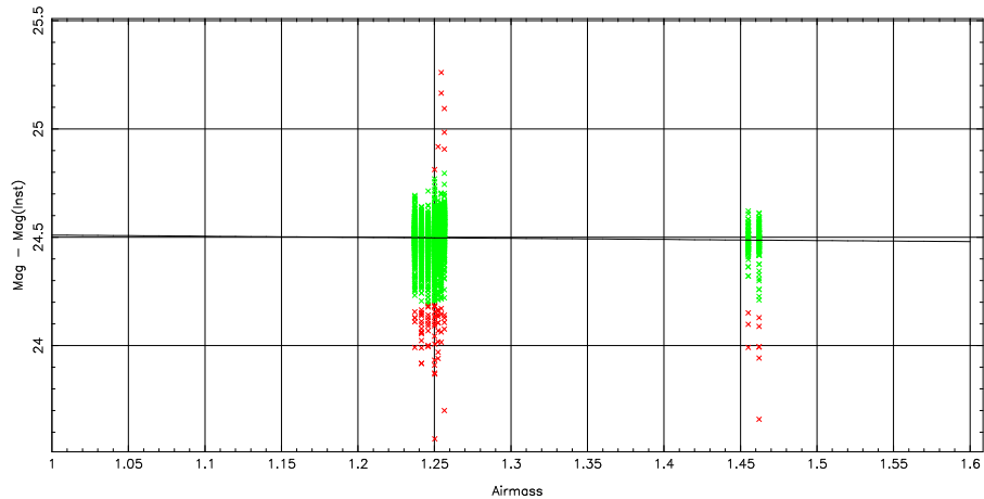
2 parameter fit: \text{Mag}-\text{Mag}(\text{Inst}) = 24.77 \pm 0.05 + (-0.22 \pm 0.00) \text{airmass} + (0.23 \pm 0.00) \text{color}
