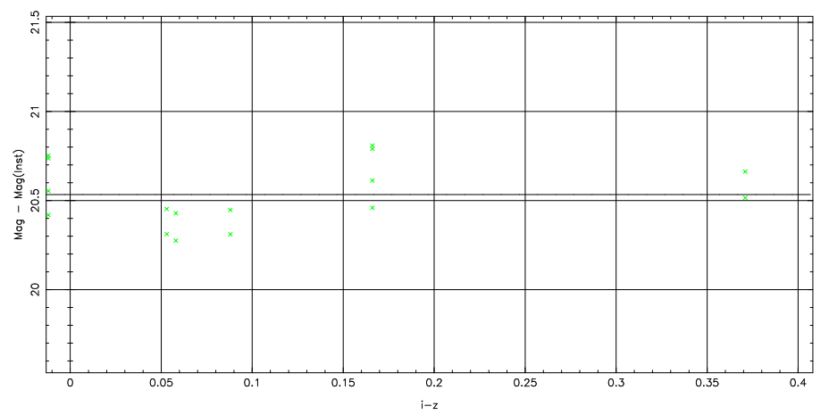
1 parameter fit: \text{Mag}-\text{Mag}(\text{Inst}) = 20.53 \pm 0.25 + (0.00 \pm 0.00) \text{airmass} + (0.00 \pm 0.00) \text{color}
