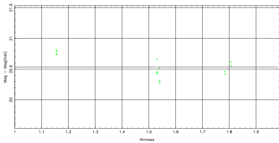
1 parameter fit: \text{Mag}-\text{Mag}(\text{Inst}) = 20.53 \pm 0.25 + (0.00 \pm 0.00) \text{airmass} + (0.00 \pm 0.00) \text{color}
