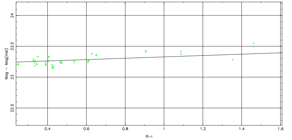
1 parameter fit: \text{Mag}-\text{Mag}(\text{Inst}) = 23.22 \pm 0.15 + (-0.10 \pm 0.00) \text{airmass} + (0.11 \pm 0.00) \text{color}
