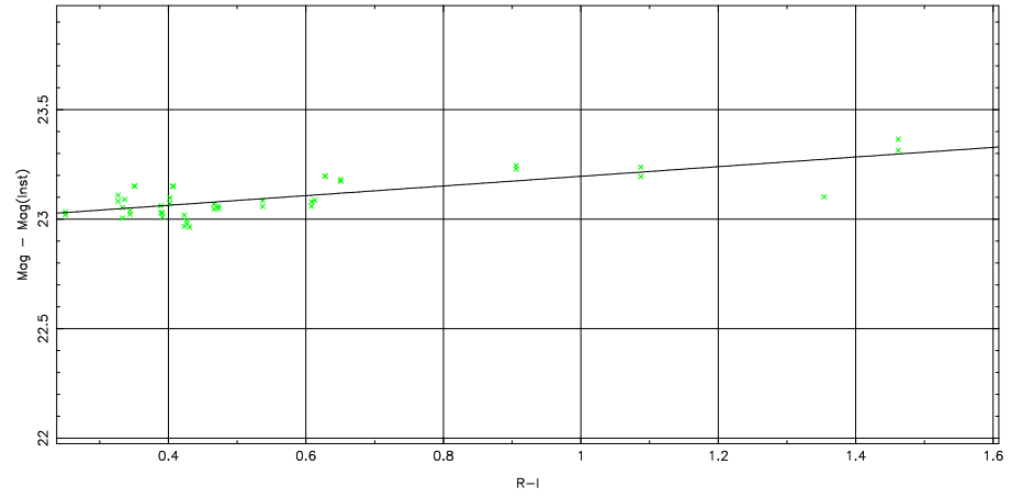
2 parameter fit: \text{Mag}-\text{Mag}(\text{Inst}) = 23.16 \pm 0.31 + (-0.10 \pm 0.00) \text{airmass} + (0.22 \pm 0.00) \text{color}
