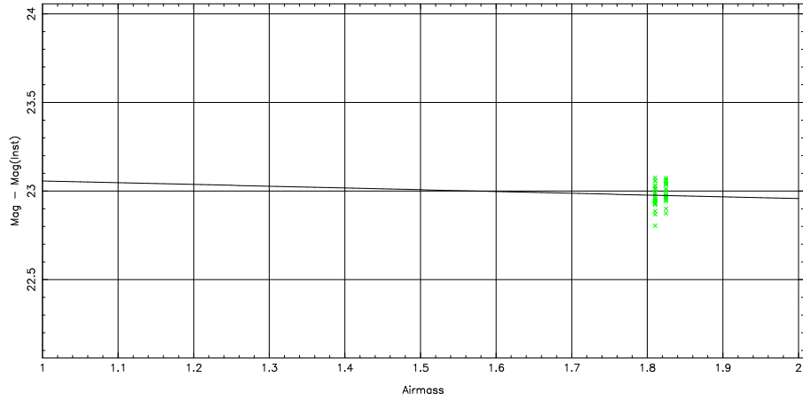
1 parameter fit: \text{Mag}-\text{Mag}(\text{Inst}) = 23.22 \pm 0.15 + (-0.10 \pm 0.00) \text{airmass} + (0.11 \pm 0.00) \text{color}
