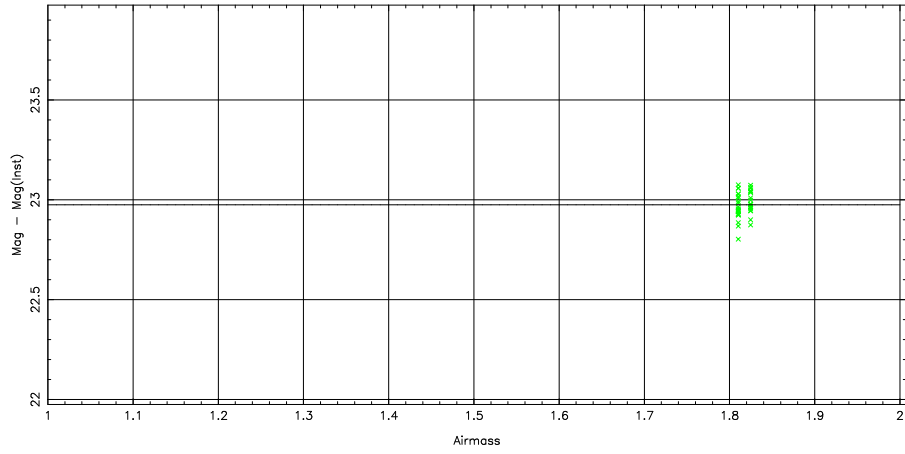
2 parameter fit: \text{Mag}-\text{Mag}(\text{Inst}) = 23.16 \pm 0.31 + (-0.10 \pm 0.00) \text{airmass} + (0.22 \pm 0.00) \text{color}
