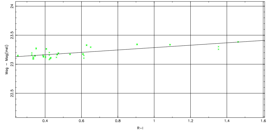
2 parameter fit: \text{Mag}-\text{Mag}(\text{Inst}) = 23.27 \pm 0.29 + (-0.10 \pm 0.00) \text{airmass} + (0.21 \pm 0.00) \text{color}
