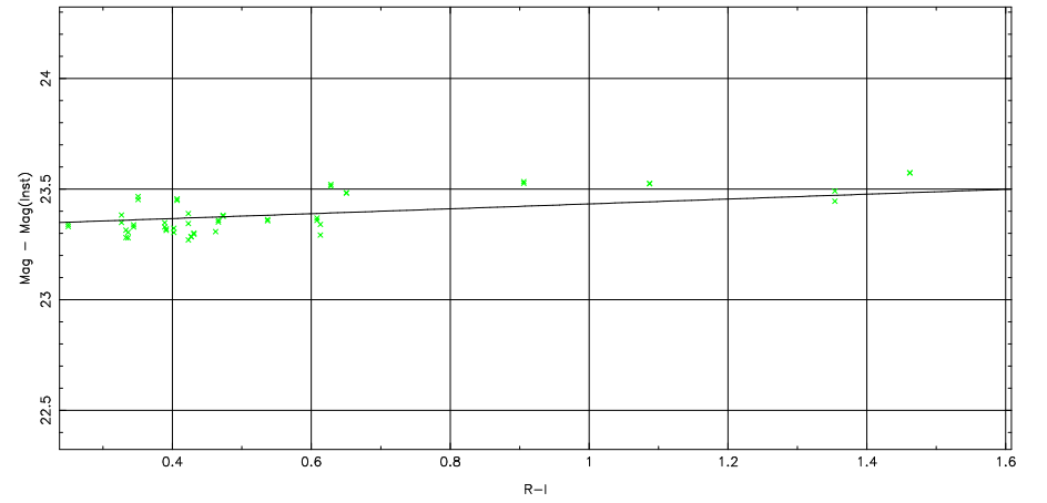
1 parameter fit: \text{Mag}-\text{Mag}(\text{Inst}) = 23.32 \pm 0.14 + (-0.10 \pm 0.00) \text{airmass} + (0.11 \pm 0.00) \text{color}
