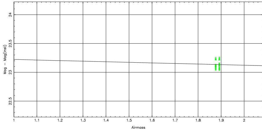
1 parameter fit: \text{Mag}-\text{Mag}(\text{Inst}) = 23.32 \pm 0.14 + (-0.10 \pm 0.00) \text{airmass} + (0.11 \pm 0.00) \text{color}
