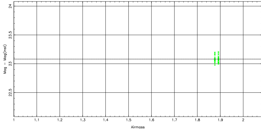
2 parameter fit: \text{Mag}-\text{Mag}(\text{Inst}) = 23.27 \pm 0.29 + (-0.10 \pm 0.00) \text{airmass} + (0.21 \pm 0.00) \text{color}
