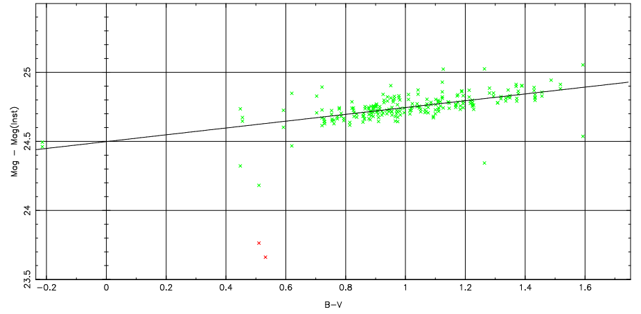
2 parameter fit: \text{Mag}-\text{Mag}(\text{Inst}) = 24.76 \pm 0.27 + (-0.22 \pm 0.00) \text{airmass} + (0.25 \pm 0.00) \text{color}
