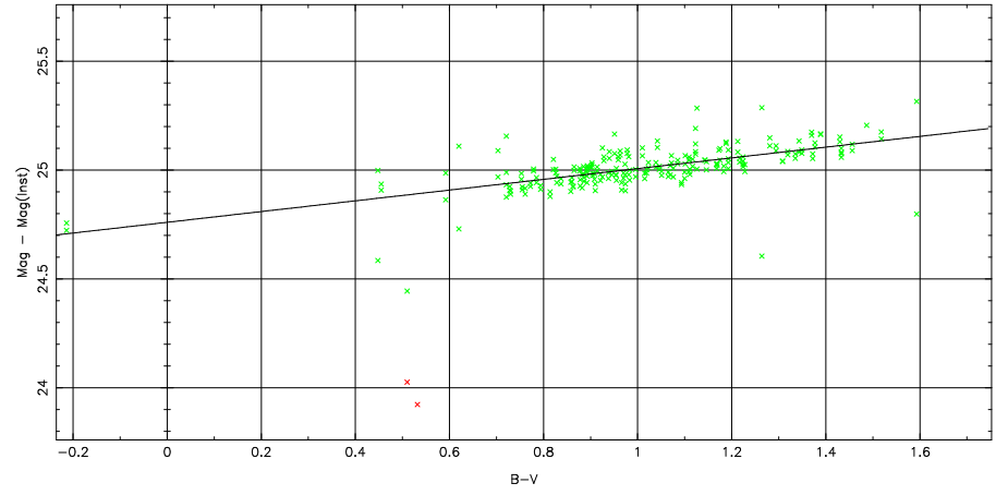
1 parameter fit: \text{Mag}-\text{Mag}(\text{Inst}) = 24.76 \pm 0.07 + (-0.22 \pm 0.00) \text{airmass} + (0.25 \pm 0.00) \text{color}
