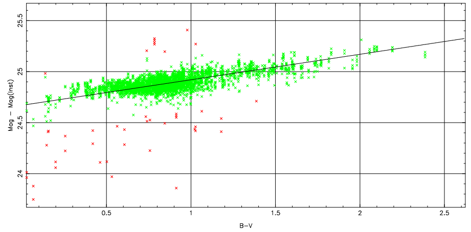
1 parameter fit: \text{Mag}-\text{Mag}(\text{Inst}) = 24.67 \pm 0.02 + (-0.22 \pm 0.00) \text{airmass} + (0.25 \pm 0.00) \text{color}
