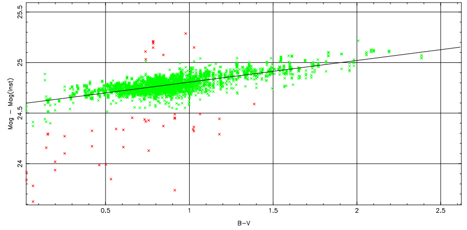
2 parameter fit: \text{Mag}-\text{Mag}(\text{Inst}) = 24.70 \pm 0.05 + (-0.22 \pm 0.00) \text{airmass} + (0.21 \pm 0.00) \text{color}
