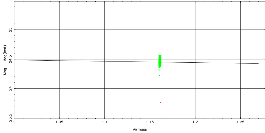
1 parameter fit: \text{Mag}-\text{Mag}(\text{Inst}) = 24.68 \pm 0.08 + (-0.22 \pm 0.00) \text{airmass} + (0.25 \pm 0.00) \text{color}
