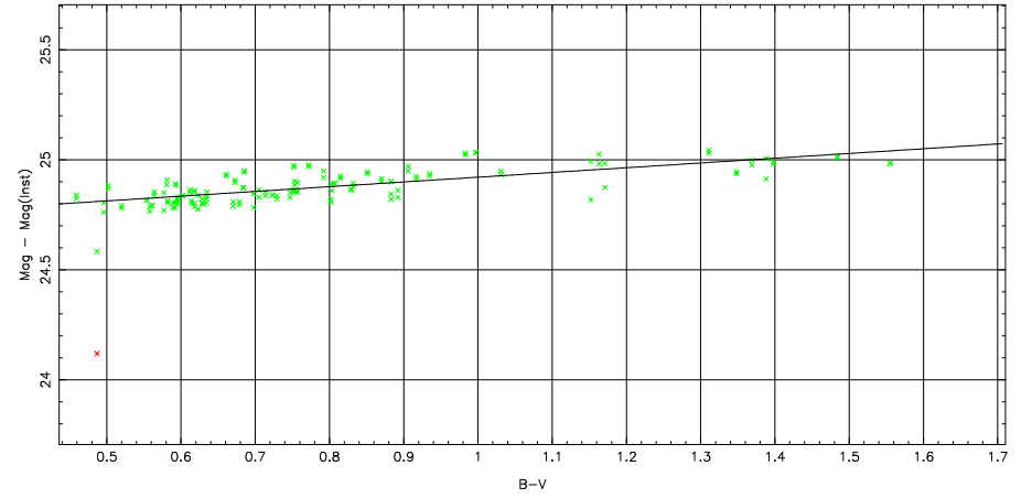
1 parameter fit: \text{Mag}-\text{Mag}(\text{Inst}) = 24.68 \pm 0.08 + (-0.22 \pm 0.00) \text{airmass} + (0.25 \pm 0.00) \text{color}
