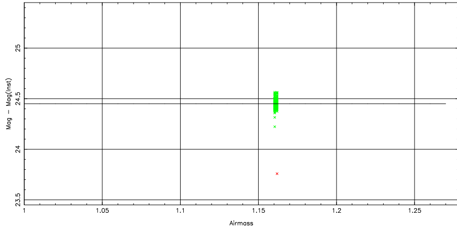
2 parameter fit: \text{Mag}-\text{Mag}(\text{Inst}) = 24.71 \pm 0.27 + (-0.22 \pm 0.00) \text{airmass} + (0.22 \pm 0.00) \text{color}
