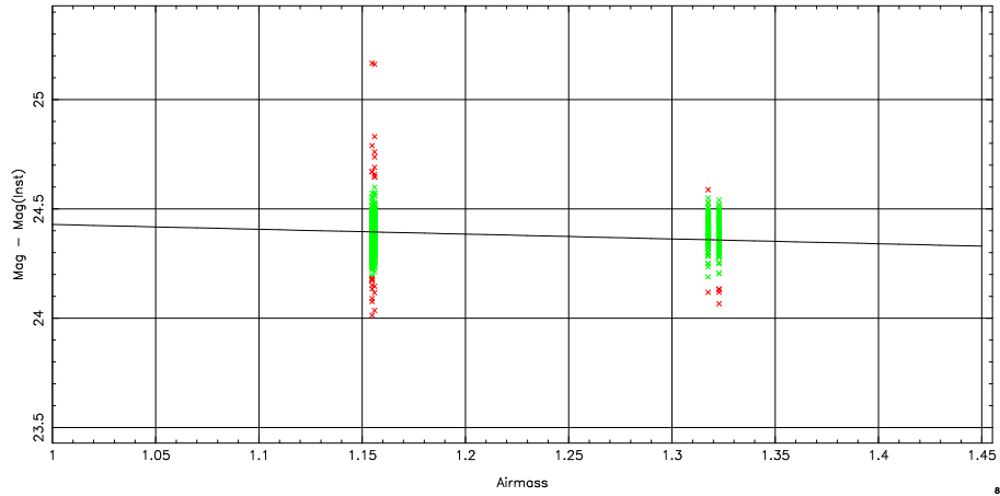
1 parameter fit: \text{Mag}-\text{Mag}(\text{Inst}) = 24.65 \pm 0.02 + (-0.22 \pm 0.00) \text{airmass} + (0.25 \pm 0.00) \text{color}
