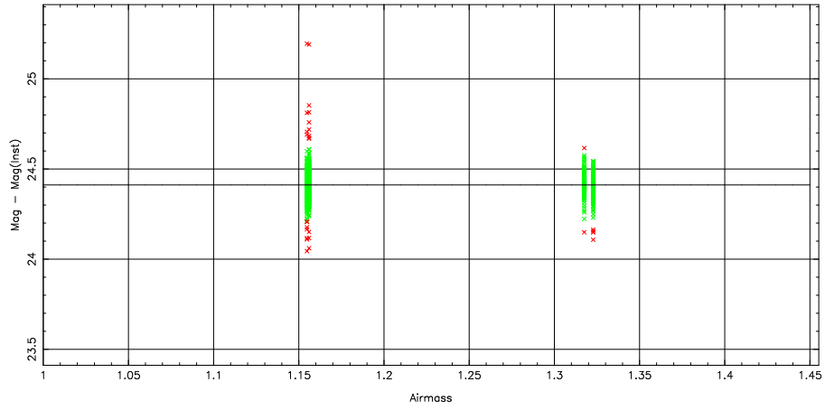
2 parameter fit: \text{Mag}-\text{Mag}(\text{Inst}) = 24.68 \pm 0.07 + (-0.22 \pm 0.00) \text{airmass} + (0.22 \pm 0.00) \text{color}
