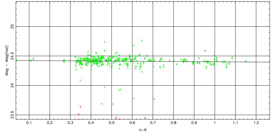
2 parameter fit: \text{Mag}-\text{Mag}(\text{Inst}) = 24.50 \pm 0.13 + (-0.07 \pm 0.00) \text{airmass} + (-0.02 \pm 0.00) \text{color}
