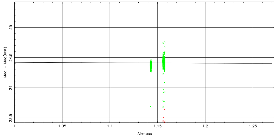
1 parameter fit: \text{Mag}-\text{Mag}(\text{Inst}) = 24.49 \pm 0.05 + (-0.07 \pm 0.00) \text{airmass} + (0.00 \pm 0.00) \text{color}
