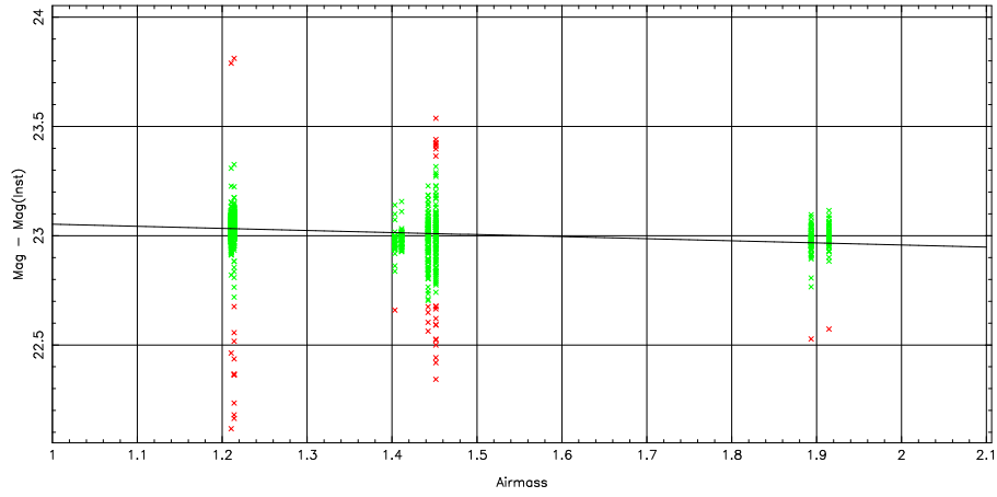
2 parameter fit: \text{Mag}-\text{Mag}(\text{Inst}) = 23.15 \pm 0.07 + (-0.10 \pm 0.00) \text{airmass} + (0.23 \pm 0.00) \text{color}
