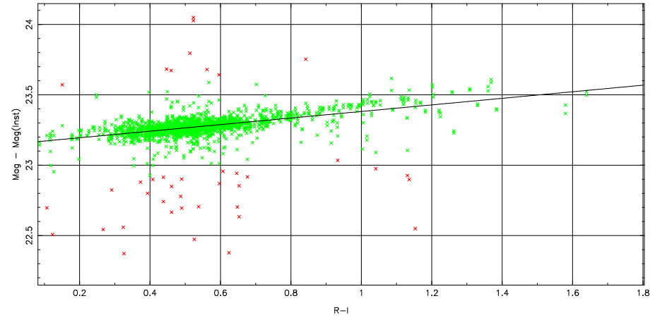
2 parameter fit: \text{Mag}-\text{Mag}(\text{Inst}) = 23.15 \pm 0.07 + (-0.10 \pm 0.00) \text{airmass} + (0.23 \pm 0.00) \text{color}
