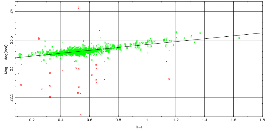
2 parameter fit: \text{Mag}-\text{Mag}(\text{Inst}) = 23.13 \pm 0.08 + (-0.10 \pm 0.00) \text{ airmass} + (0.25 \pm 0.00) \text{ color}
