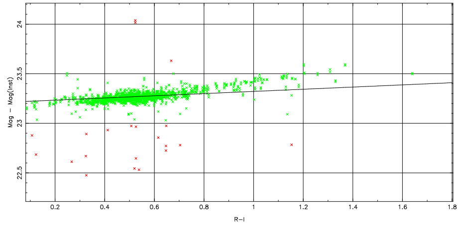
1 parameter fit: \text{Mag}-\text{Mag}(\text{Inst}) = 23.21 \pm 0.03 + (-0.10 \pm 0.00) \text{ airmass} + (0.11 \pm 0.00) \text{ color}
