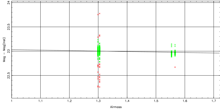
1 parameter fit: \text{Mag}-\text{Mag}(\text{Inst}) = 23.21 \pm 0.03 + (-0.10 \pm 0.00) \text{ airmass} + (0.11 \pm 0.00) \text{ color}
