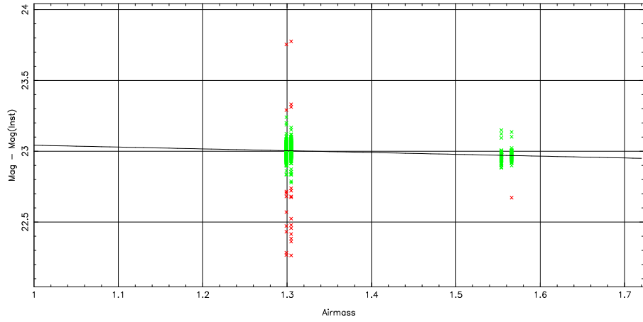
2 parameter fit: \text{Mag}-\text{Mag}(\text{Inst}) = 23.13 \pm 0.08 + (-0.10 \pm 0.00) \text{ airmass} + (0.25 \pm 0.00) \text{ color}
