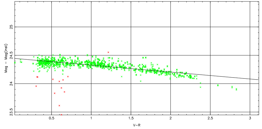
2 parameter fit: \text{Mag}-\text{Mag}(\text{Inst}) = 24.55 \pm 0.07 + (-0.07 \pm 0.00) \text{airmass} + (-0.11 \pm 0.00) \text{color}
