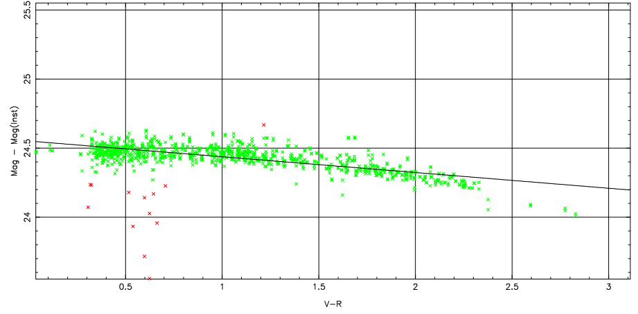
1 parameter fit: \text{Mag}-\text{Mag}(\text{Inst}) = 24.43 \pm 0.03 + (-0.07 \pm 0.00) \text{airmass} + (0.00 \pm 0.00) \text{color}
