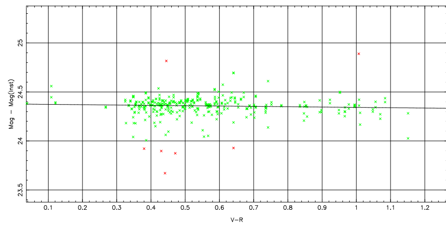
2 parameter fit: \text{Mag}-\text{Mag}(\text{Inst}) = 24.46 \pm 0.16 + (-0.07 \pm 0.00) \text{airmass} + (-0.03 \pm 0.00) \text{color}
