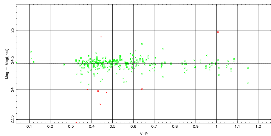
1 parameter fit: \text{Mag}-\text{Mag}(\text{Inst}) = 24.44 \pm 0.05 + (-0.07 \pm 0.00) \text{airmass} + (0.00 \pm 0.00) \text{color}
