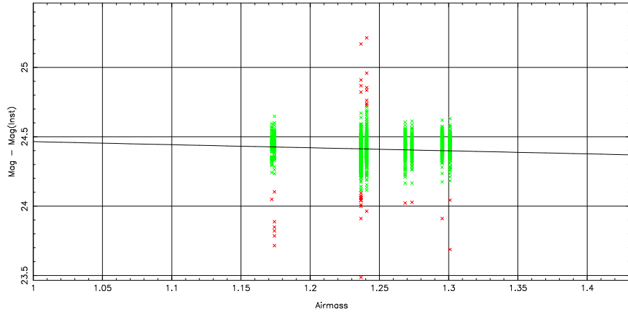
1 parameter fit: \text{Mag}-\text{Mag}(\text{Inst}) = 24.66 \pm 0.02 + (-0.22 \pm 0.00) \text{airmass} + (0.25 \pm 0.00) \text{color}
