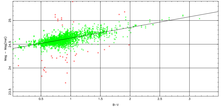
2 parameter fit: \text{Mag}-\text{Mag}(\text{Inst}) = 24.69 \pm 0.06 + (-0.22 \pm 0.00) \text{airmass} + (0.22 \pm 0.00) \text{color}
