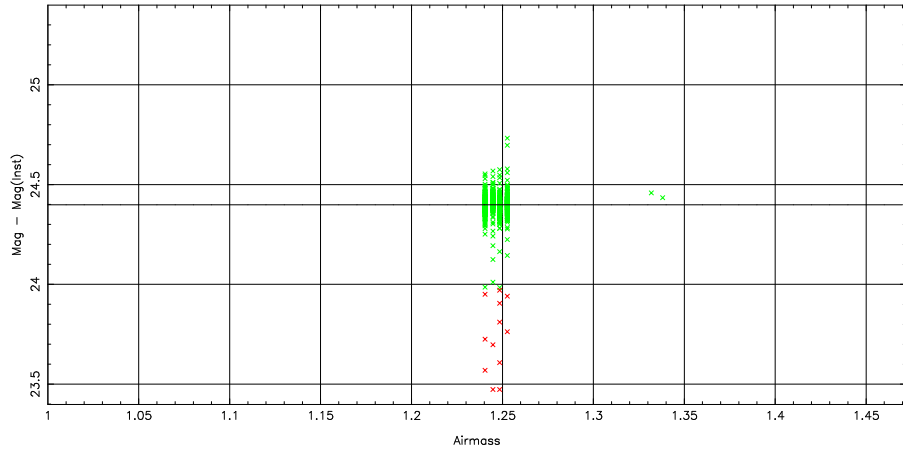
2 parameter fit: \text{Mag}-\text{Mag}(\text{Inst}) = 24.49 \pm 0.11 + (-0.07 \pm 0.00) \text{airmass} + (-0.04 \pm 0.00) \text{color}
