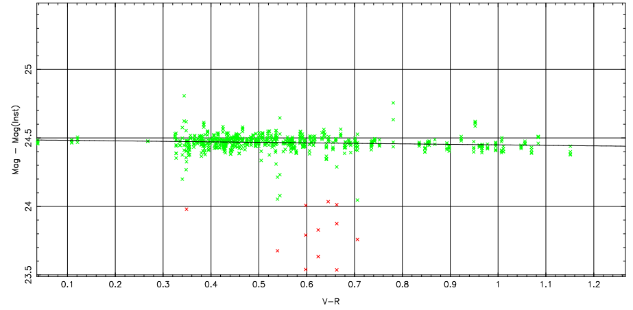
1 parameter fit: \text{Mag}-\text{Mag}(\text{Inst}) = 24.47 \pm 0.04 + (-0.07 \pm 0.00) \text{airmass} + (0.00 \pm 0.00) \text{color}
