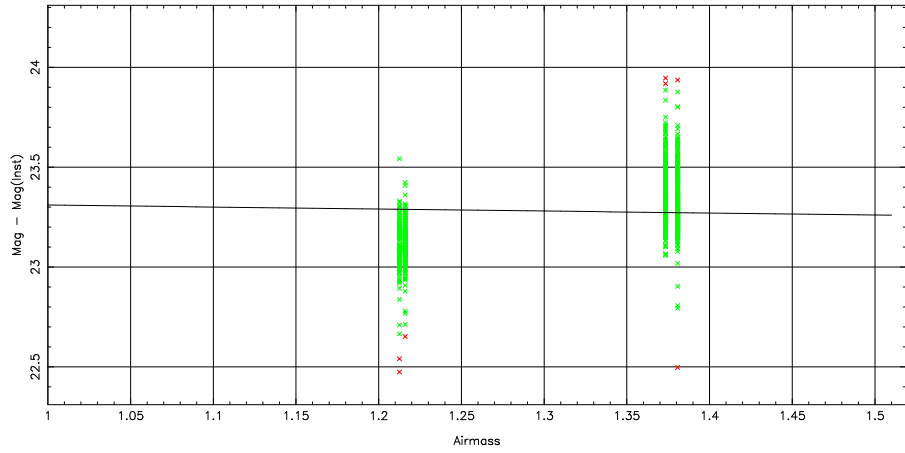
1 parameter fit: \text{Mag}-\text{Mag}(\text{Inst}) = 23.41 \pm 0.03 + (-0.10 \pm 0.00) \text{airmass} + (0.11 \pm 0.00) \text{color}
