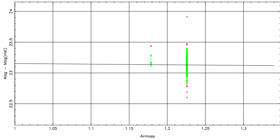
1 parameter fit: \text{Mag}-\text{Mag}(\text{Inst}) = 23.25 \pm 0.04 + (-0.10 \pm 0.00) \text{ airmass} + (0.11 \pm 0.00) \text{ color}
