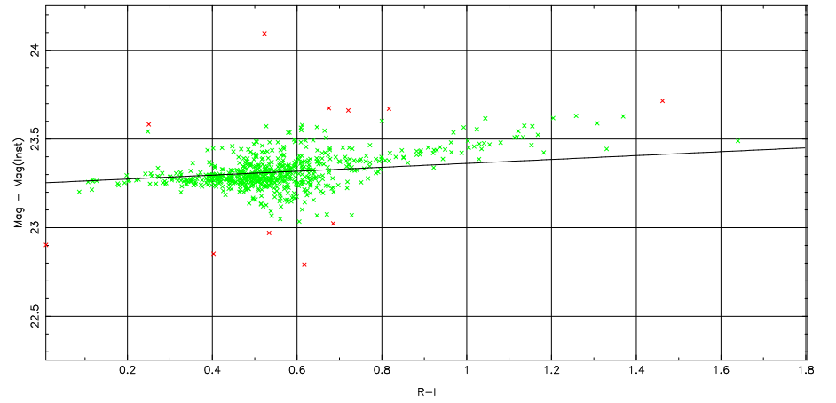
1 parameter fit: \text{Mag}-\text{Mag}(\text{Inst}) = 23.25 \pm 0.04 + (-0.10 \pm 0.00) \text{ airmass} + (0.11 \pm 0.00) \text{ color}
