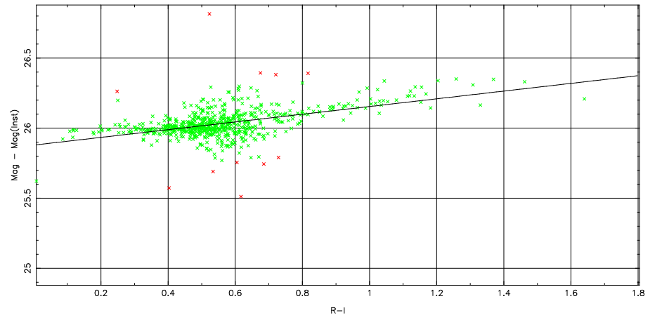
2 parameter fit: \text{Mag}-\text{Mag}(\text{Inst}) = 23.16 \pm 0.12 + (-0.10 \pm 0.00) \text{ airmass} + (0.28 \pm 0.00) \text{ color}
